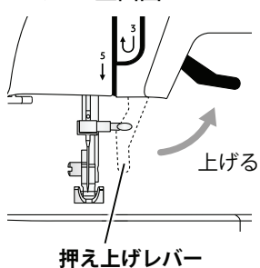
< ミシン正面図 >
